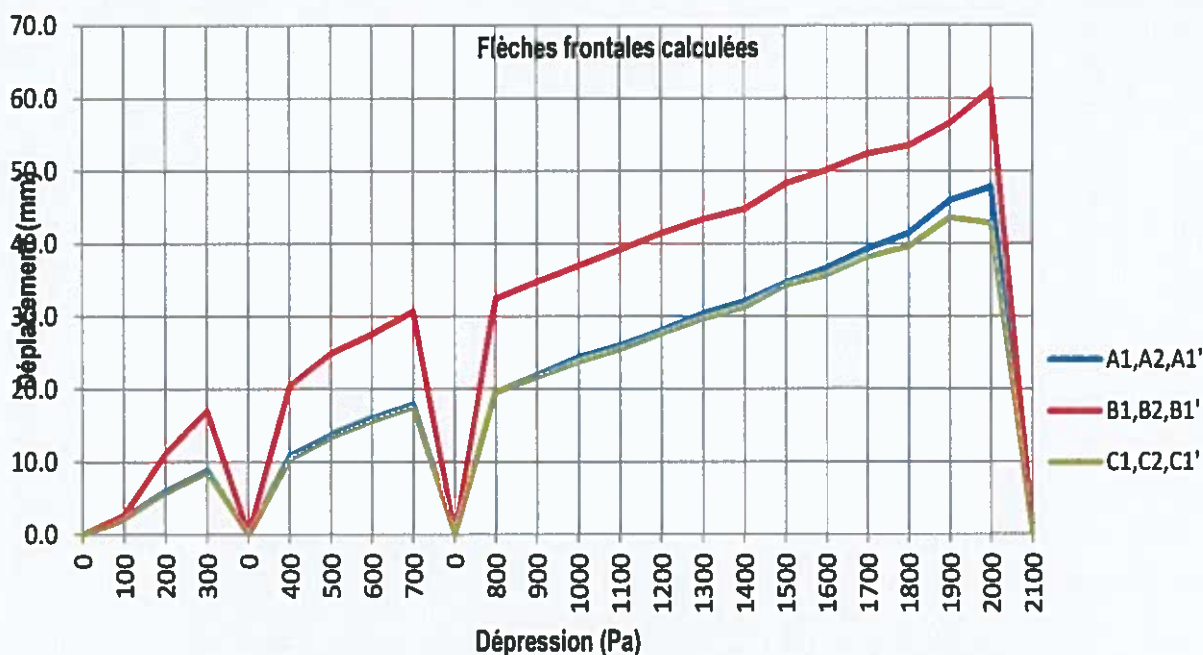
Grphe n°4 : Flèches frontales calculées en dépression
