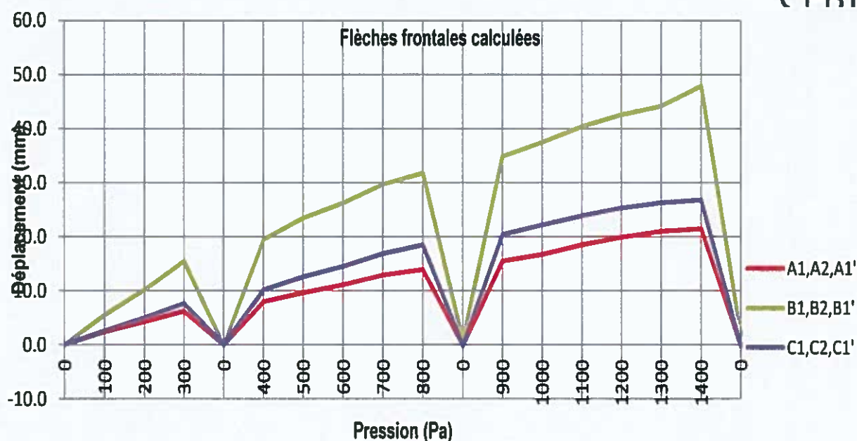
Graphe n°2 : Flèches frontales calculées en pression
