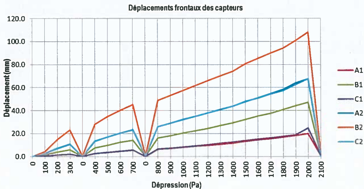
Graphe n° 3 : Déplacements frontaux mesurés en dépression
